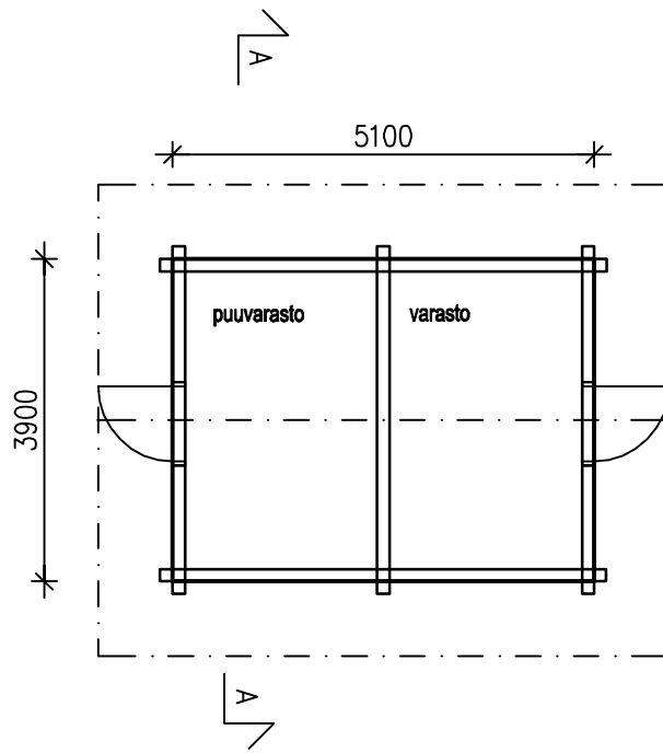
Varaston pohja 1:100
