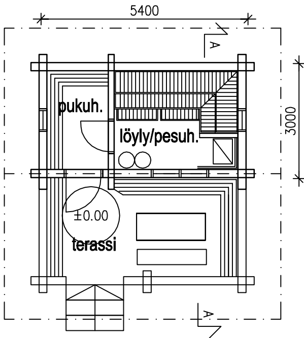
Saunarakennus pohja 1:100
