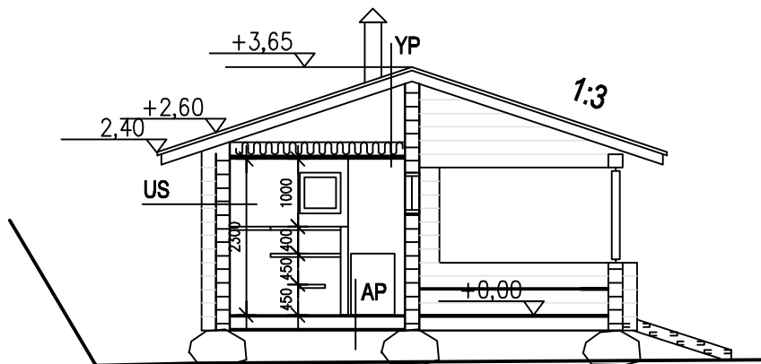
Leikkaus A-A
